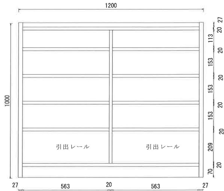
内面図
