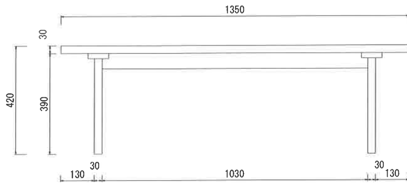
正面図
