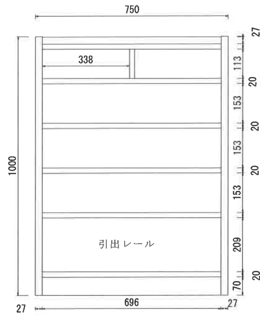
内面図
