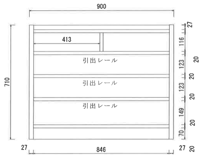
内面図
