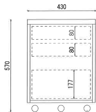
内面図
