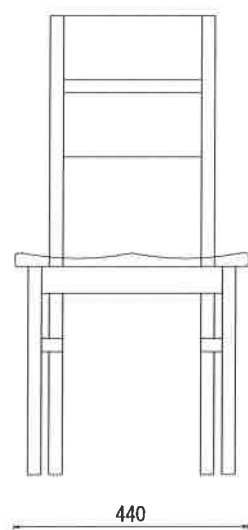
正面図
