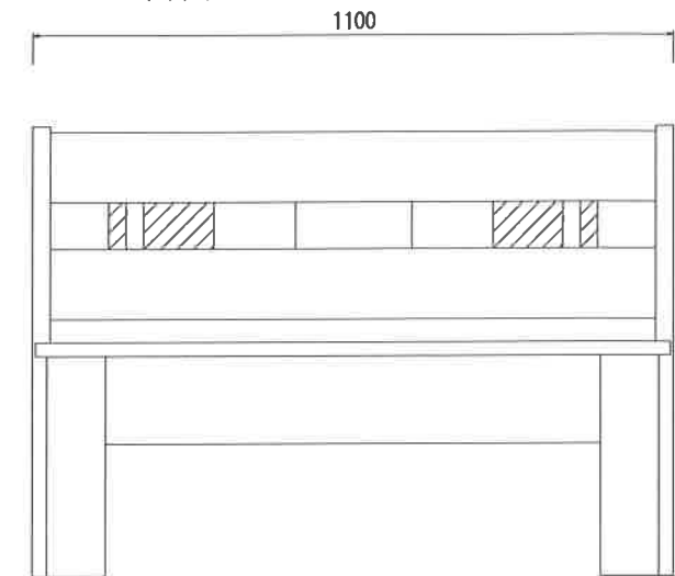
正面図
