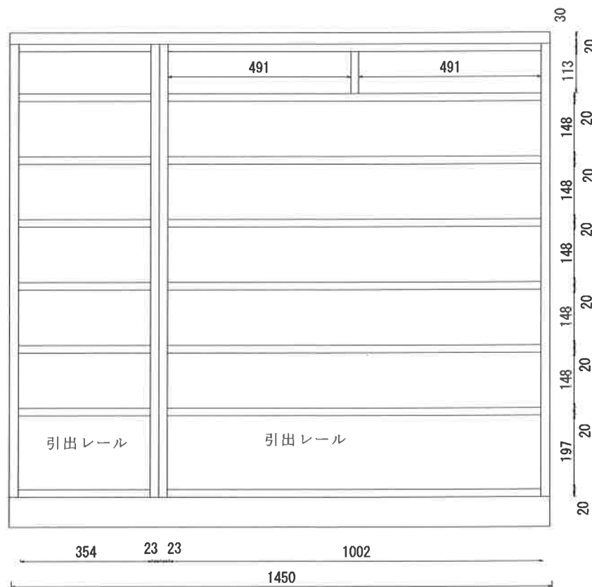
内面図
