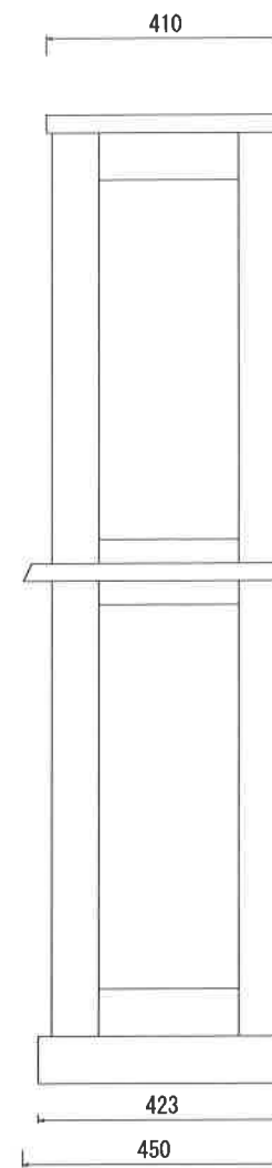
断面図
