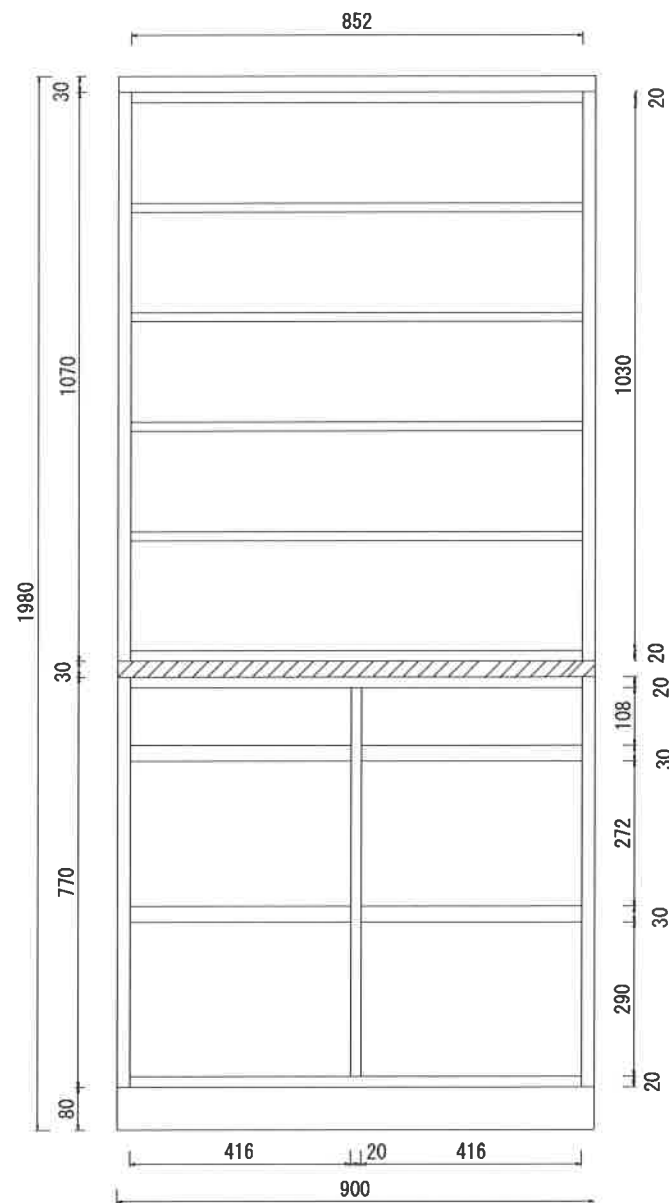
内面図
