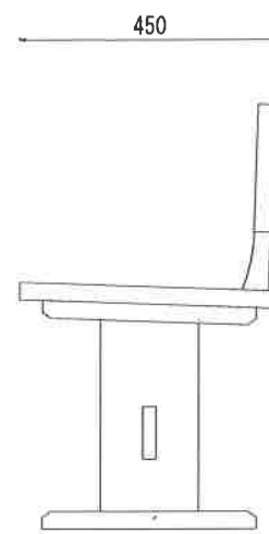
断面図
