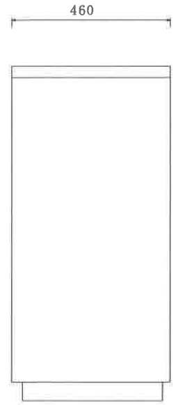
断面図
