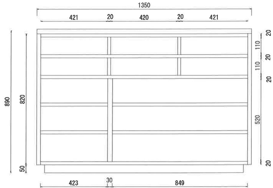
内面図
