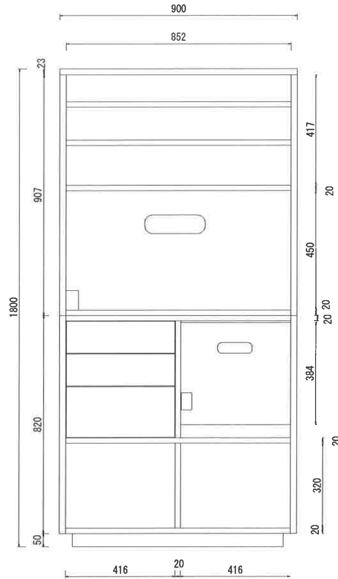
内面図
