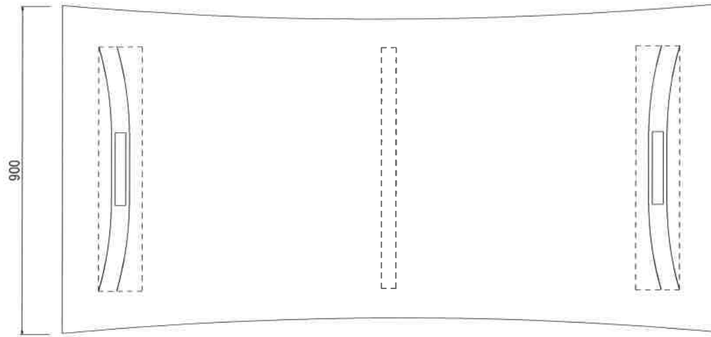
正面図
